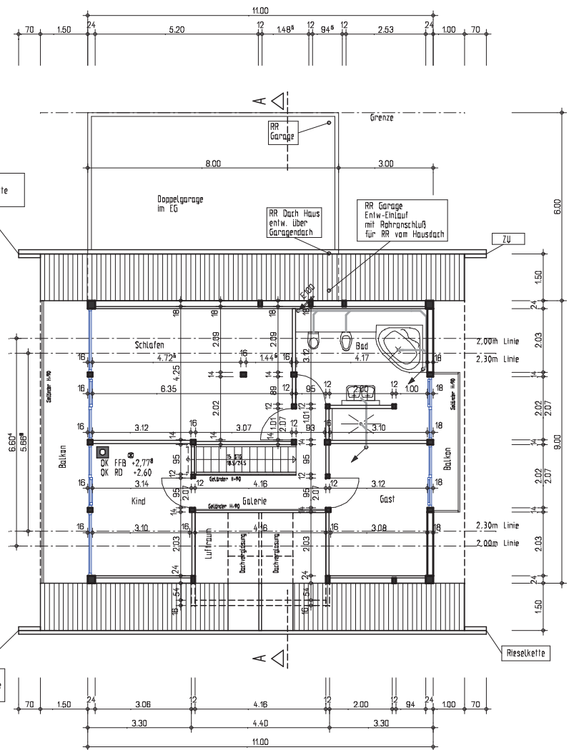
Grundriss Dachgeschoß
