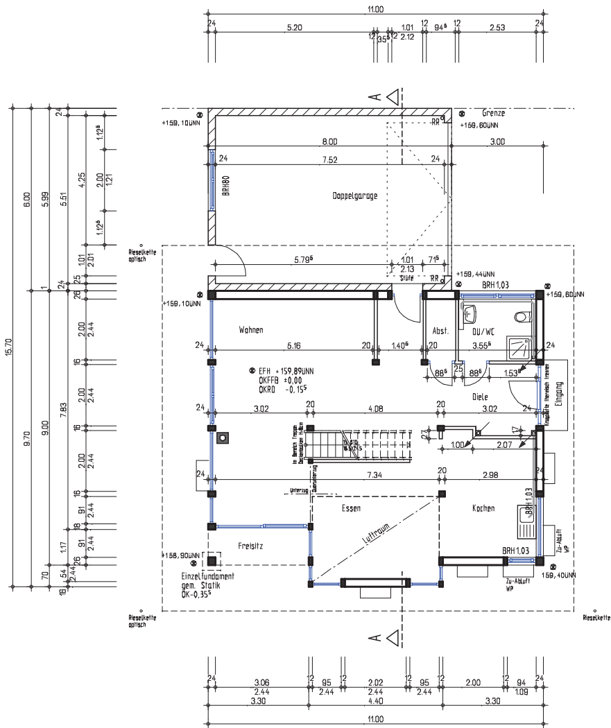
Grundriss Erdgeschoß
