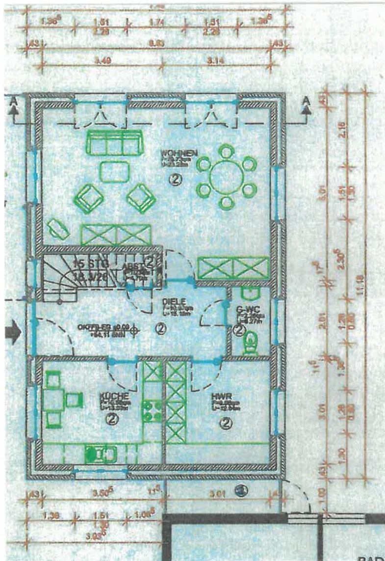
ERDGESCHOSS
