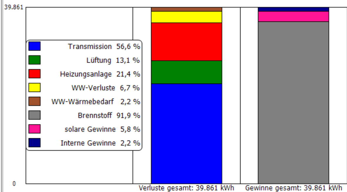
Jährliche Energieverluste und -gewinne
