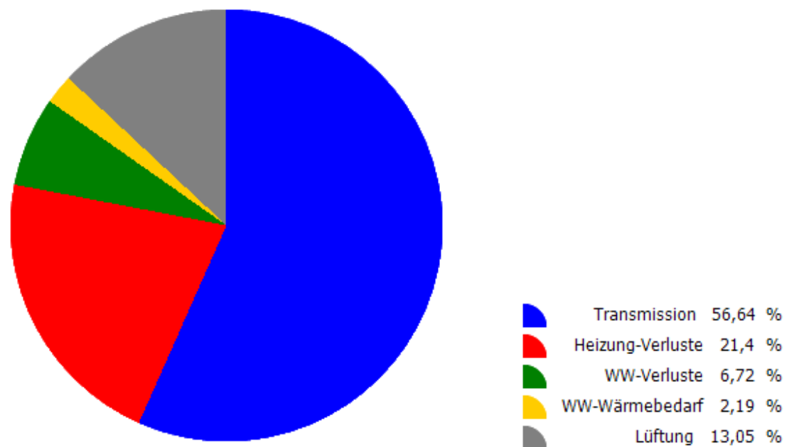
Jährliche Verluste in Prozent
