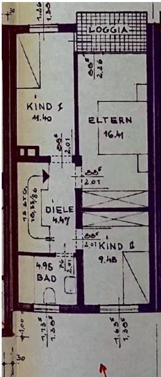
Oberschoss
