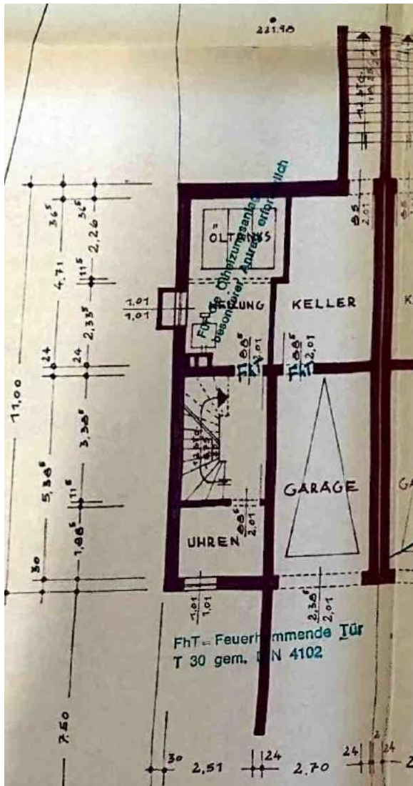
Kellergeschoss
